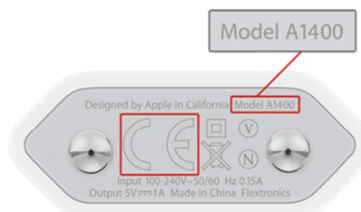
Adaptador redesenhado
